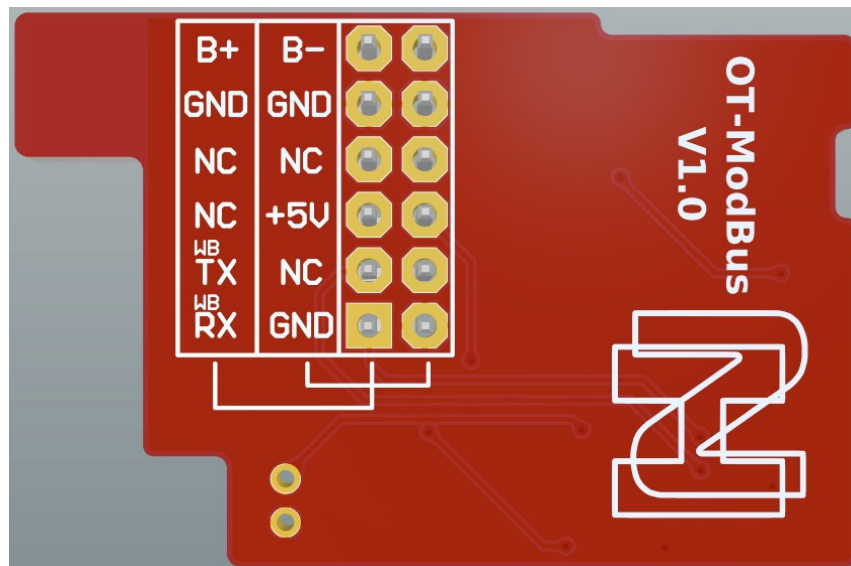
Рисунок 2 – Вид снизу.
